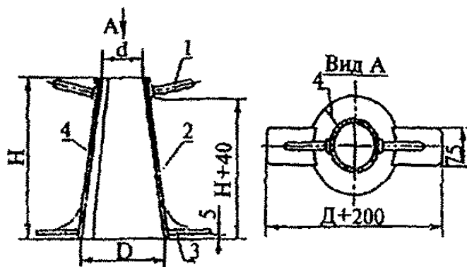
1 - ручка; 2 - корпус; 3 - упоры; 4 - сварной шов.
