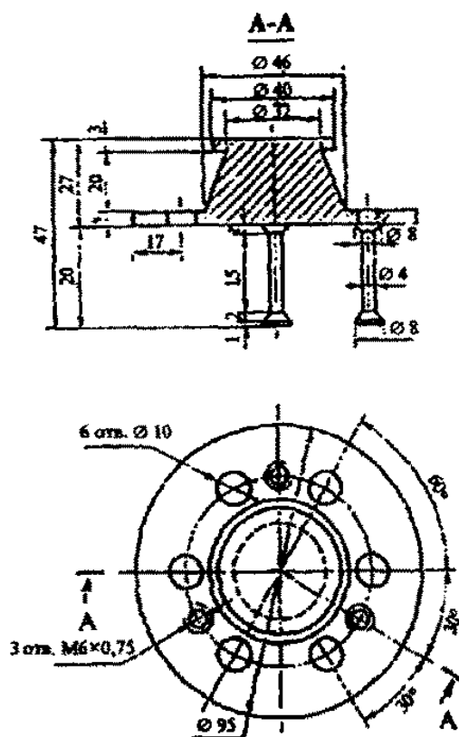
Рисунок 3 - Прибор Красного
