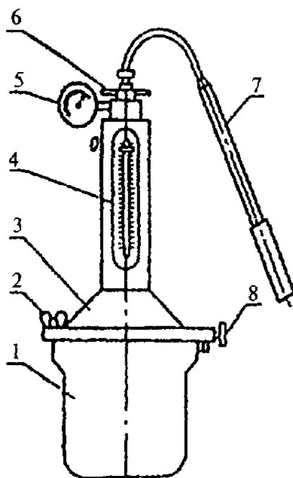
Рисунок 4 - Объёммер
